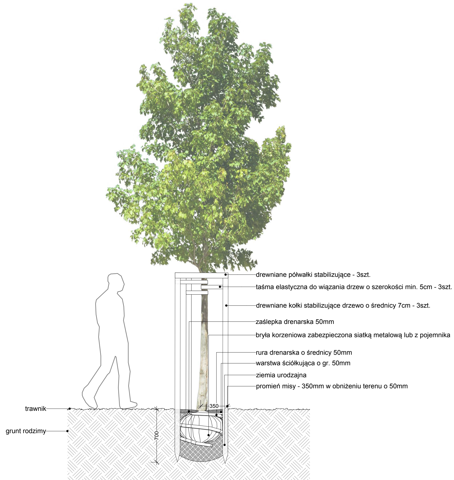
5 Detal sadzenia drzew formy piennej Skala 1:25
